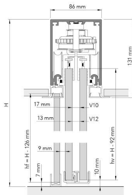
MONTAJE EMPOTRADO CON VIDRIO FIJO
