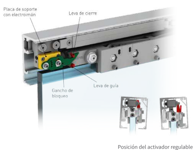
Posición del activador regulable
