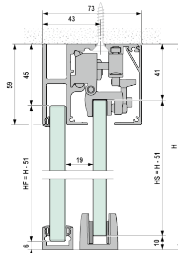
MONTAJE A TECHO CON HOJA FIJA
