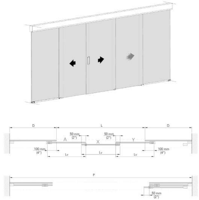
Extendo 3 hojas con vidrio fijo
