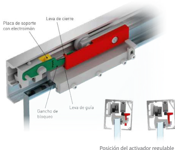
Posición del activador regulable
