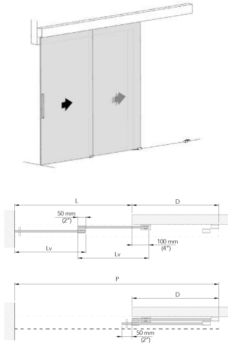
Extendo 2 hojas sin vidrio fijo
