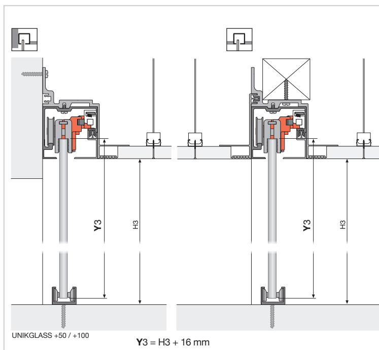
MONTAJE EMPOTRADO CON DINTEL
