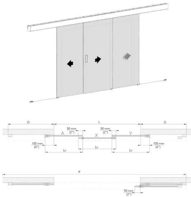
Extendo 3 hojas sin vidrio fijo
