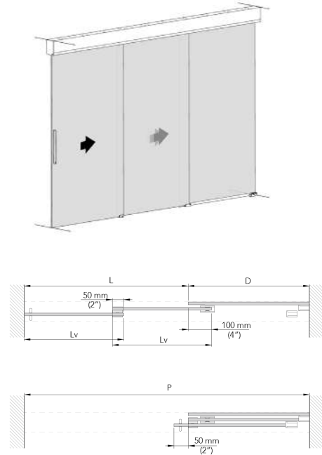
Extendo 2 hojas con vidrio fijo
