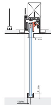
UNIKGLASS + EMPOTRADO SIN DINTEL
