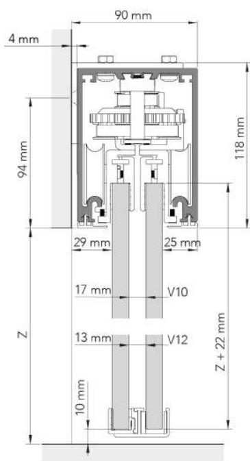
MONTAJE VISTO SIN VIDRIO FIJO
