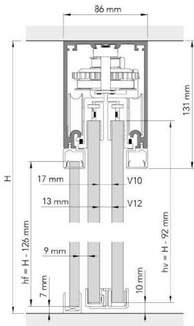
MONTAJE VISTO CON VIDRIO FIJO
